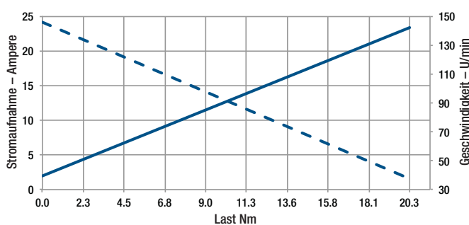
K2RAG30-12VDC
