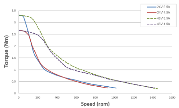
NEMA 23 Long (IP20, IP65)
