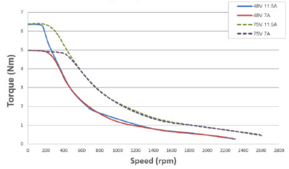
NEMA 34 Medium (IP65)
