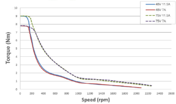
NEMA 34 Long (IP65)
