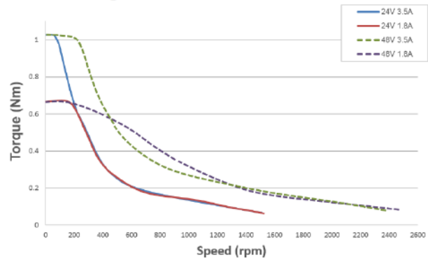
NEMA 17 Long (IP20)
